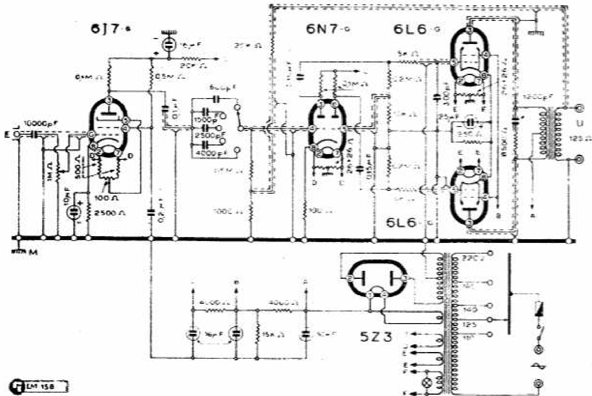
Allocchio Bacchini Amplificatore mod 1516
